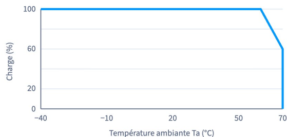
Charge selon la température ambiante (montage horizontal)
