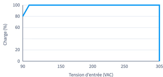
Charge selon la tension d'entrée (60 Hz)
