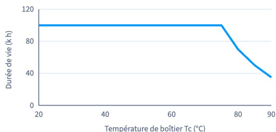
Durée de vie selon la température de boîtier Tc
