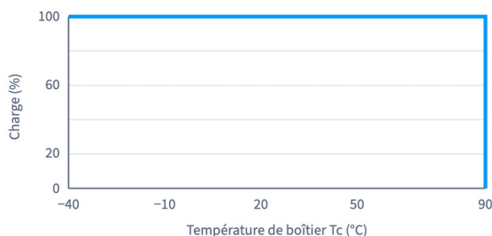
Charge selon la température de boîtier Tc
